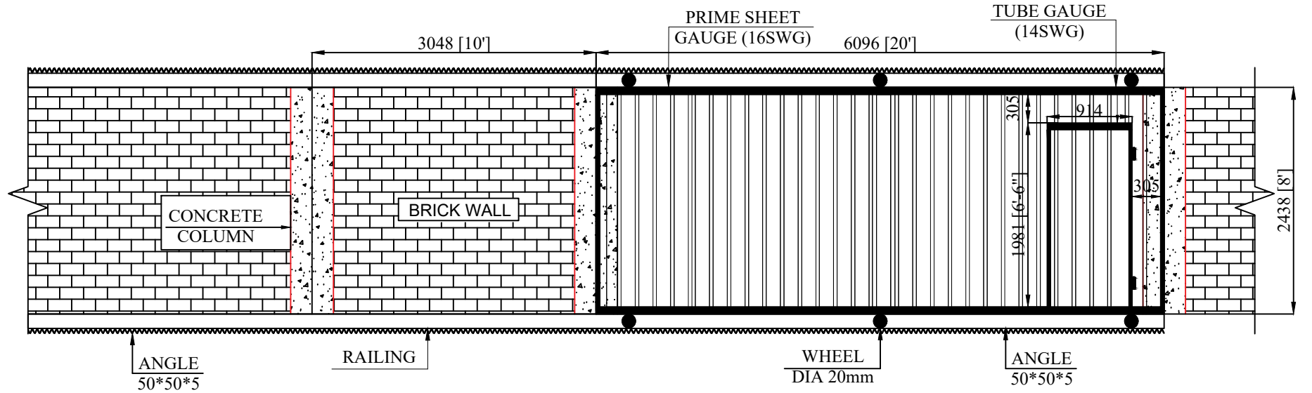
DOOR ELEVATION
